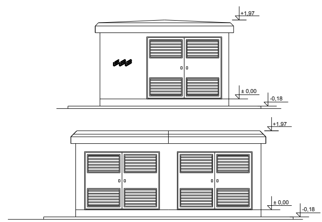
EBB KTS3 2x630(2x1000) kVA, 10/0,4kV
