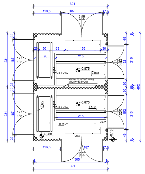
EBB KTS3 2x630(2x1000) kVA, 10/0,4kV
